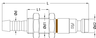
Plugs / Nippel
